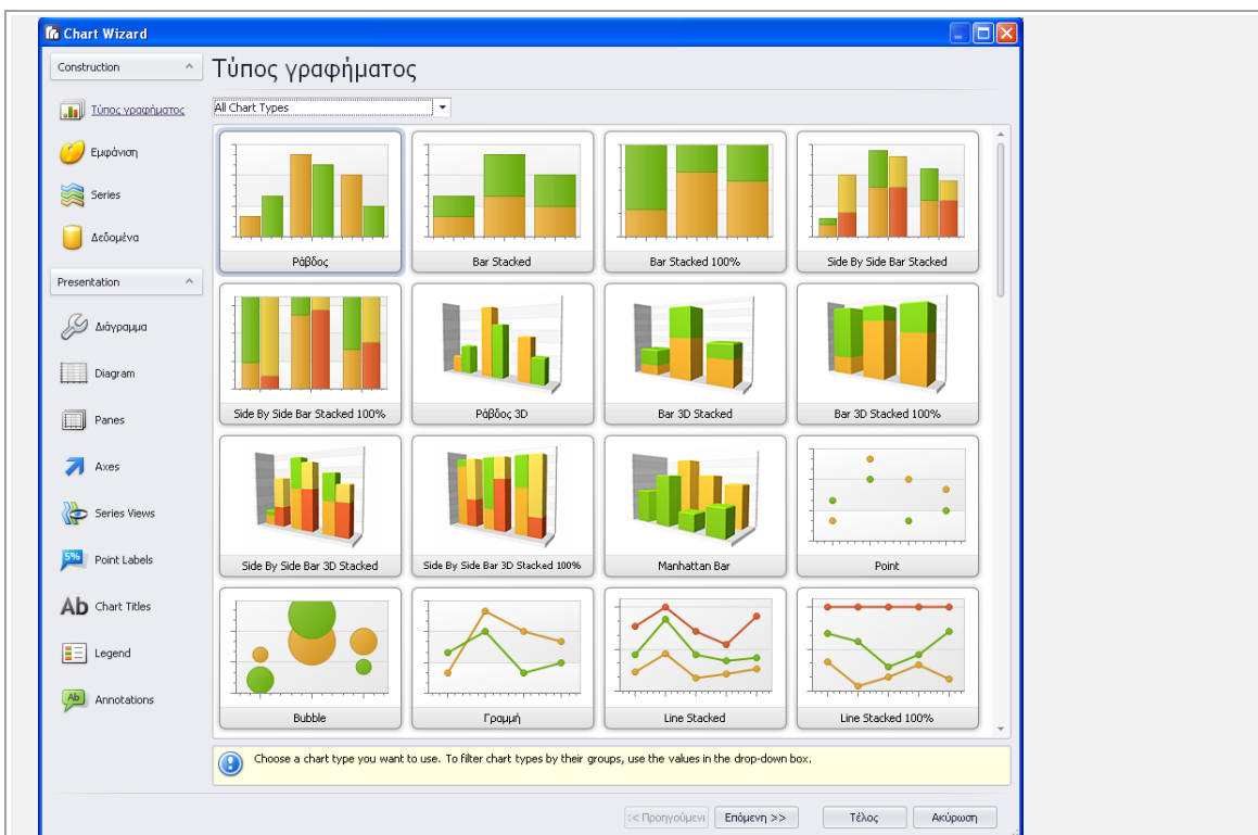
Σχήμα 1.1.5.1 Τύπος γραφήματος
