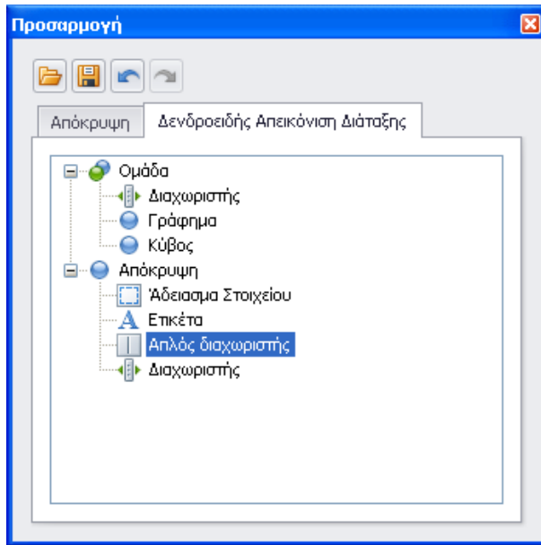
Σχήμα 1.2.1.4a Μεταβολή Layout
