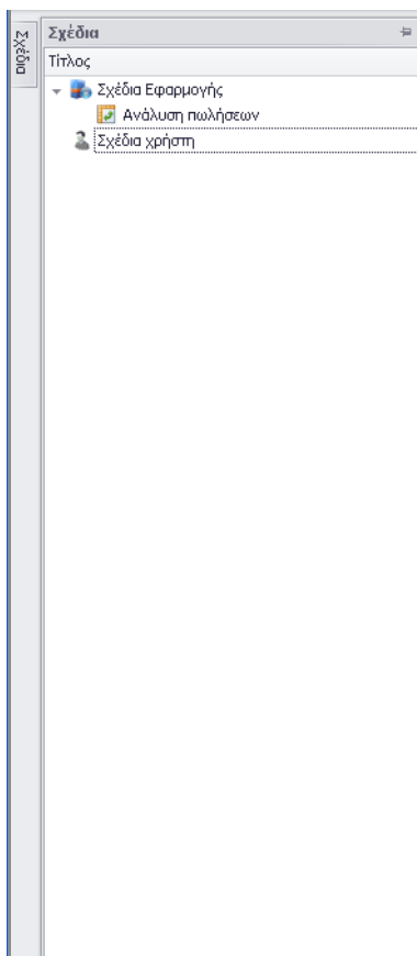
Σχήμα 1.1.2.3.1 Λίστα Σχεδίων
